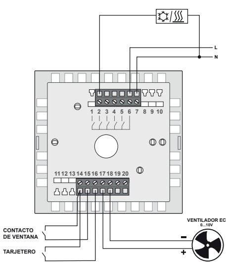
ESQUEMA 2: Fan-coil 2 tubos con cambio frío/calor local Regulación sobre válvula y ventilador EC (cont-auto)
