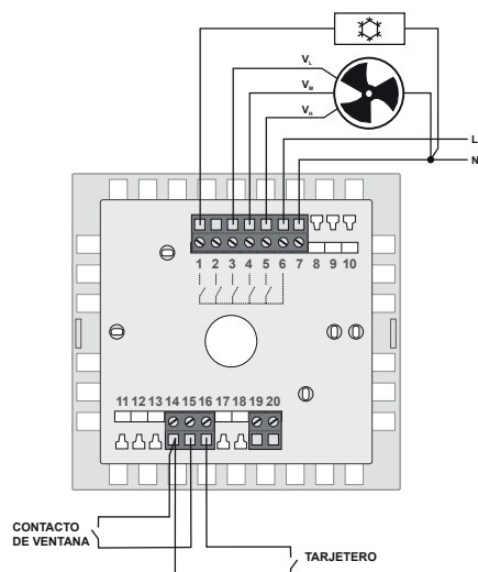
ESQUEMA 1: Fan-coil 2 tubos solo frío
