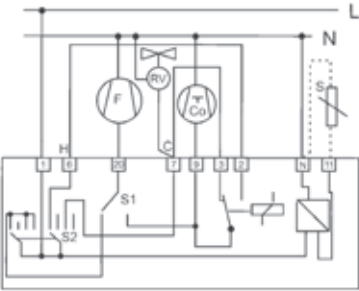
ESQUEMA 2: Bomba de calor reversible con válvula inversora energizada en refrigeración. Ventilador continuo/automático. Solamente es aplicable para aquellas máquinas en las que exista una maniobra específica para energizar la válvula inversora y permitan mantenerla energizada permanentemente cuando se selecciona el modo de funcionamiento de refrigeración.
