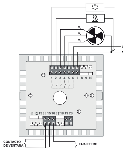
ESQUEMA 3: Fan-coil 4 tubos con cambio frío/calor automático
