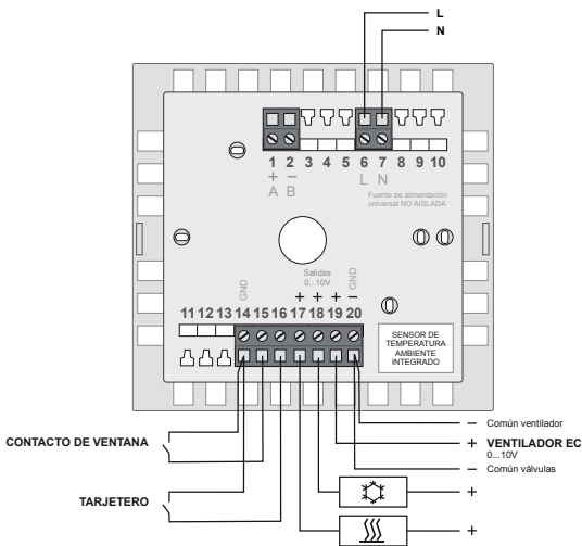
ESQUEMA 3: Fan-coil 4 tubos con cambio frío/calor automático
