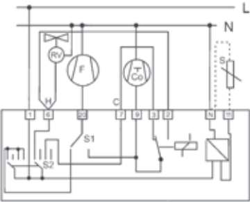
ESQUEMA 1: Bomba de calor reversible con válvula inversora energizada en calefacción. Ventilador continuo/automático. Solamente es aplicable para aquellas máquinas en las que exista una maniobra específica para energizar la válvula inversora y permitan mantenerla energizada permanentemente cuando se selecciona el modo de funcionamiento de calefacción.
