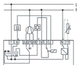
ESQUEMA 4: Fan-coil a cuatro tubos. Regulación sobre válvula y mando sobre ventilador. La selección frío o calor se realiza en el selector del propio termostato.
