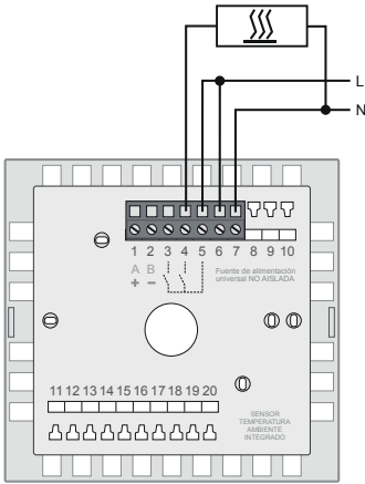
ESQUEMA 2: Regulación solo calor
