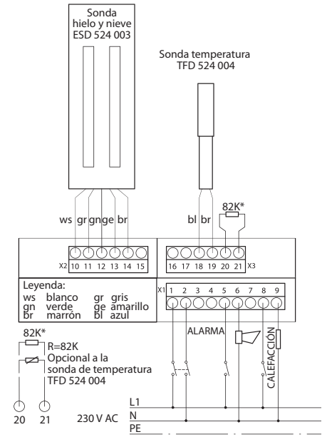
Esquema de conexión de la central de hielo y nieve con las sondas ESD 524 003 y TFD 524 004 para canales
