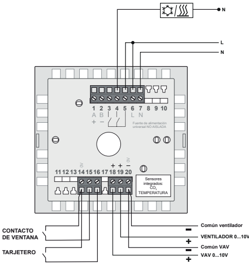
Fan-coil 2 tubos con cambio frío/calor local y compuerta VAV (CO 2 ) Regulación sobre válvula y ventilador EC (cont-auto) y compuerta VAV (CO 2 )
