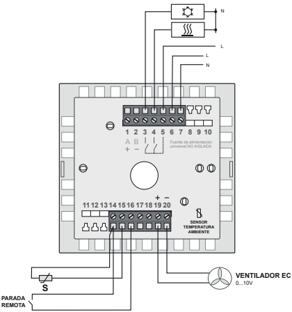
ESQUEMA 3: Fan-coil 4 tubos Regulación sobre válvula y ventilador EC (cont-auto)
