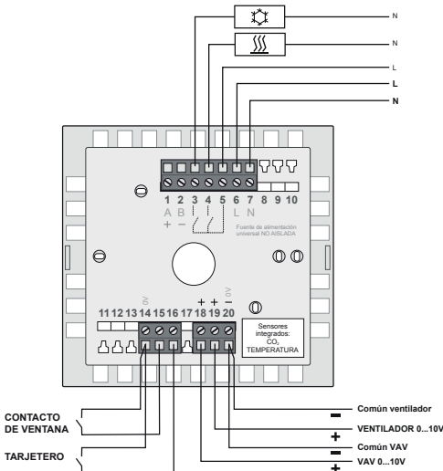
ESQUEMA 2: Fan-coil 4 tubos con cambio frío/calor automático y compuerta VAV (CO 2 ) Regulación sobre válvulas y ventilador EC (cont-auto) y compuerta VAV (CO 2 )
