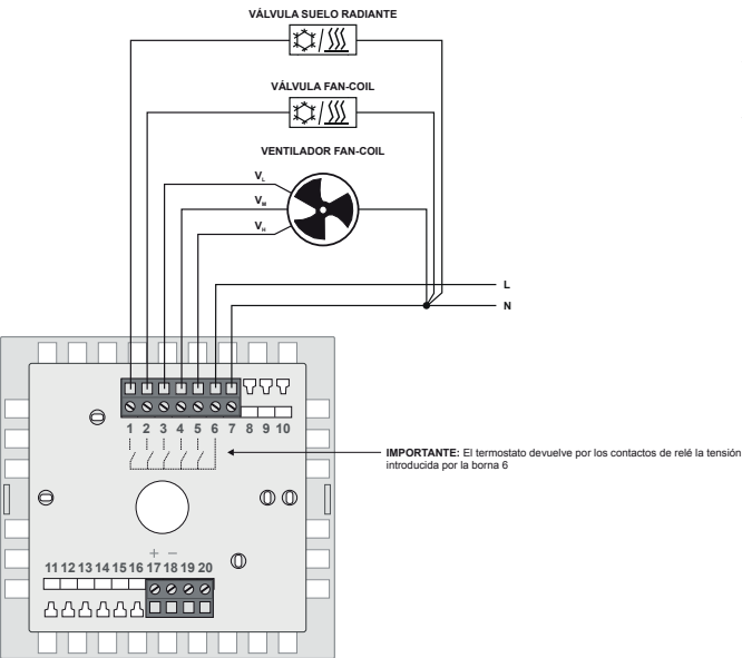
ESQUEMA 1: Suelo radiante/refrescante y fan-coil frío/calor. Regulación sobre válvula y 3 velocidades de ventilador (cont-auto)
