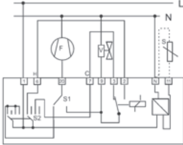
ESQUEMA 3: Fan-coil a dos tubos con cambio frío/calor local. Regulación sobre válvula. Ventilador continuo/automático.
