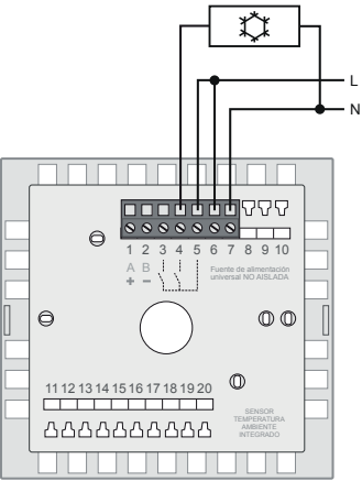
ESQUEMA 1: Regulación solo frío
