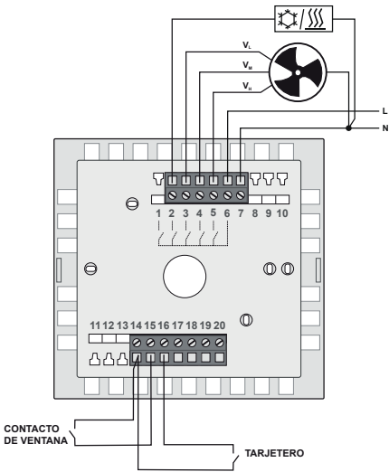
ESQUEMA 1: Fan-coil 2 tubos con cambio frío/calor local Regulación sobre válvula y 3 velocidades de ventilador (cont-auto)
