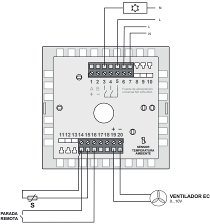
ESQUEMA 1: Fan-coil 2 tubos solo frío Regulación sobre válvula y ventilador EC (cont-auto)
