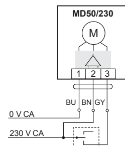
Control a 2 puntos
