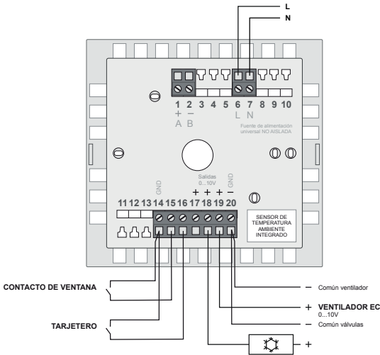
ESQUEMA 1: Fan-coil 2 tubos solo frío
