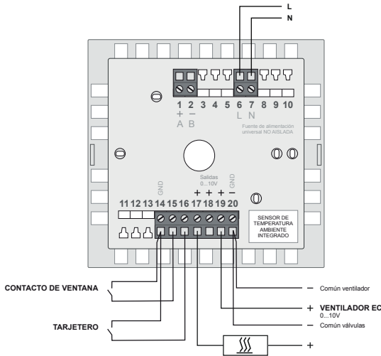
ESQUEMA 2: Fan-coil 2 tubos solo calor
