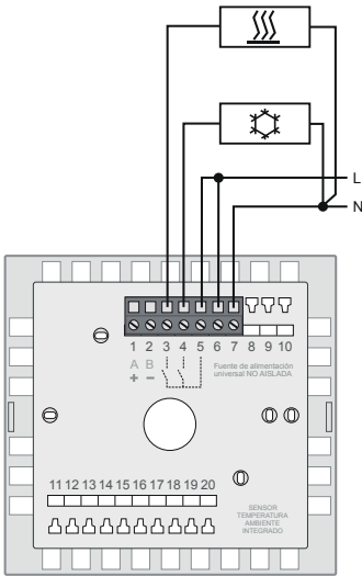
ESQUEMA 2: Regulación frío y calor
