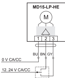
Control a 3 puntos
