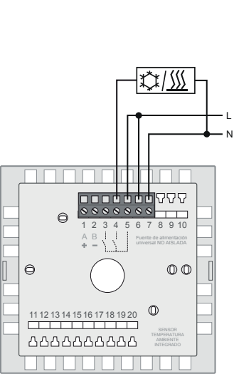
ESQUEMA 3: Regulación frío/calor
