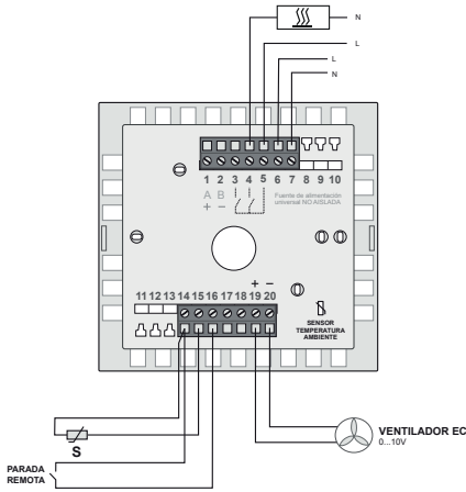
ESQUEMA 2: Fan-coil 2 tubos solo calor Regulación sobre válvula y ventilador EC (cont-auto)
