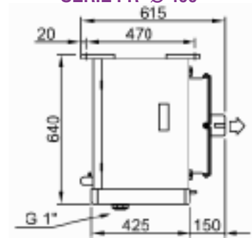
SERIE FR Ø 400
